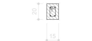
SEÇÃO A-A ESC 1:25
